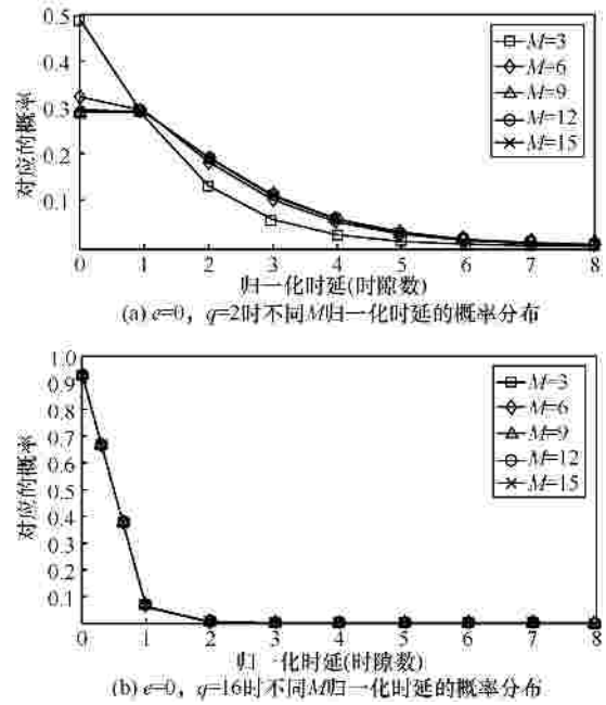
图 8 编码批次大小对时延分布的影响
