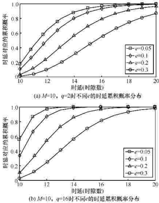
图 6 信道丢失率对时延分布的影响
