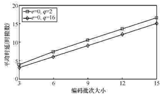
图 9 编码批次大小对平均时延的影响
